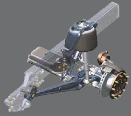
더욱 뛰어난 승차감과 전후 독립차고 조정이 가능한 전, 후륜 풀 에어서스펜션 시스템 (D38엔진 차종)
